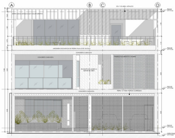
FACHADA SUR ESC. 1:50
