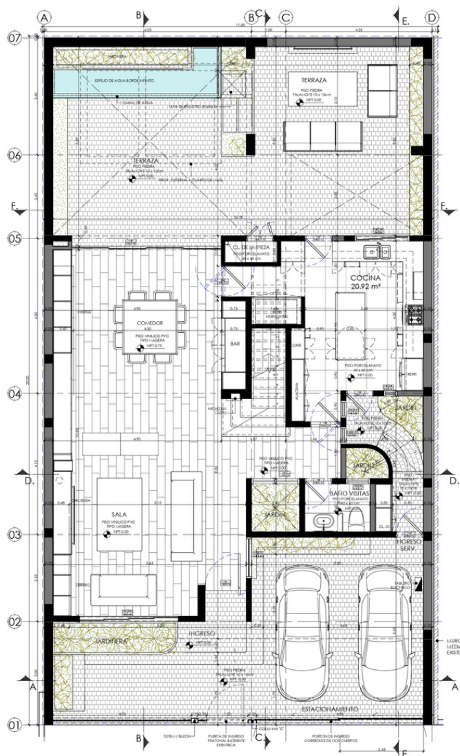
PISO 01 ESC. 1:50
