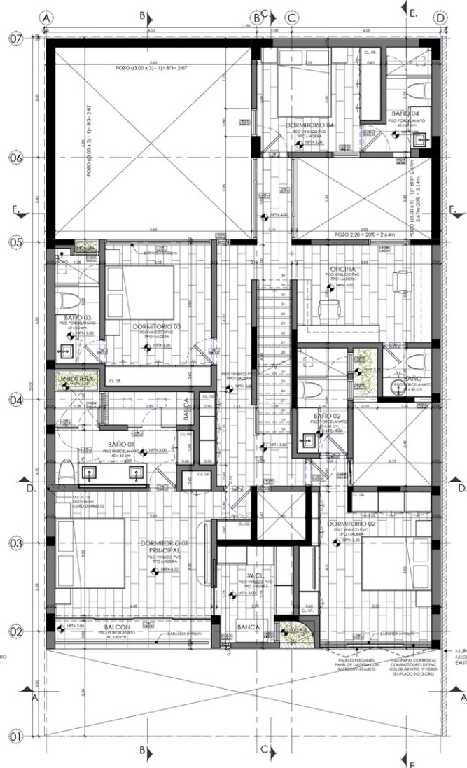
PISO 02 ESC. 1:50
